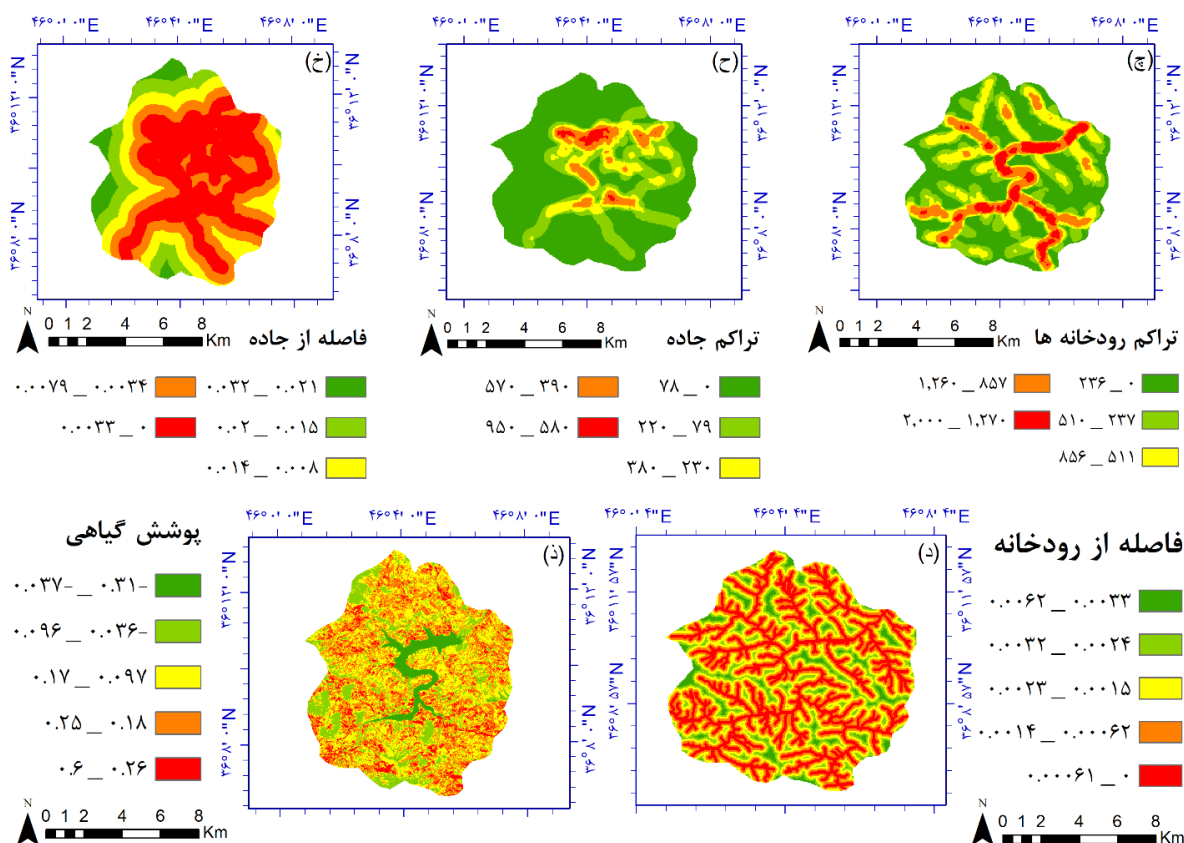
شکل ۳. تراکم رودخانه چ؛ تراکم جاده ح؛ فاصله از جاده خ؛ فاصله از رودخانه د و پوشش گیاهی ذ
